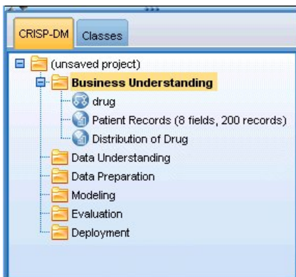
Figura 8. Visualização CRISP-DM
