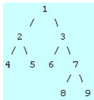
Figure 3. Exemple d'arbre de classification par division
