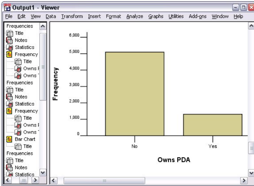
图 29: 条形图
