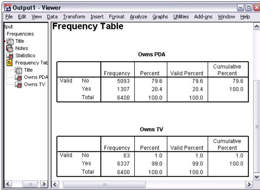
图 27: 频率表
