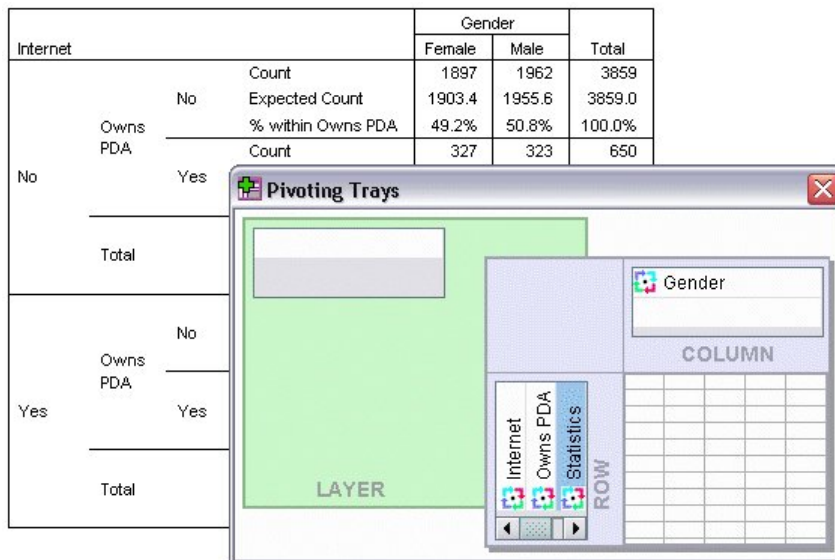
Abbildung 40. Pivot-Leisten
