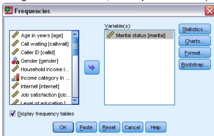
Abbildung 69. Dialogfeld "Häufigkeiten"
