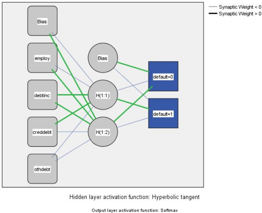
圖 1: 具有一個隱藏層的前饋架構
