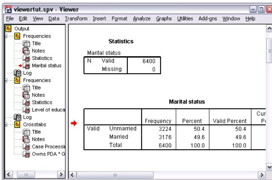
Figura 37. Visualizador
