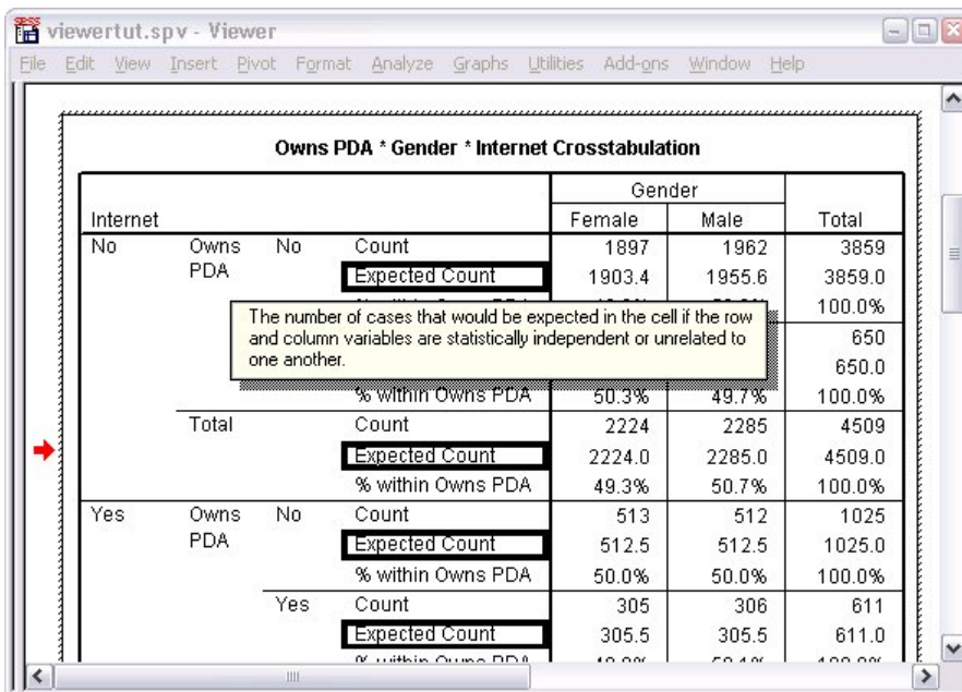
Figura 39. Definição pop-up
