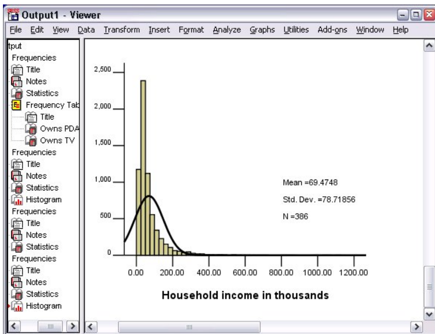
Figura 31. Histograma
