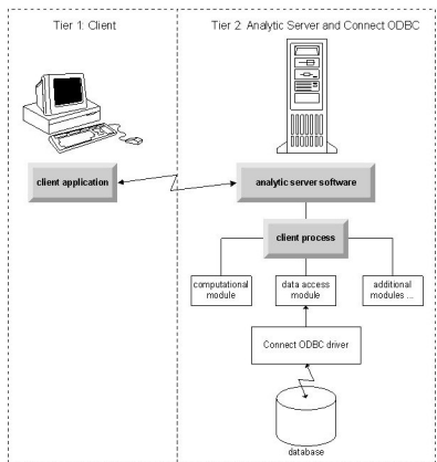
그림 3. 분산 분석 모드의 Connect ODBC
