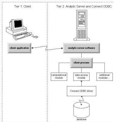
Рисунок 1. Connect ODBC в режиме распределенного анализа
