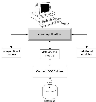
Рисунок 2. Connect ODBC в режиме локального анализа
