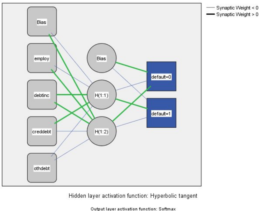
Abbildung 1. Feedforward-Architektur mit einer einzigen verborgenen Schicht
