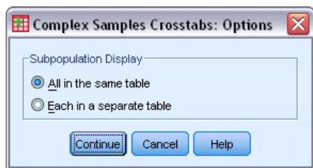
圖 5. 「選項」對話框
