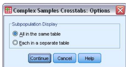
圖 8. 「選項」對話框
