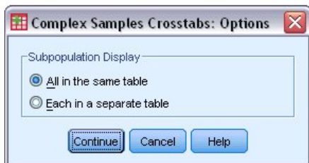
圖 4. 「選項」對話框
