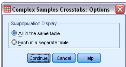
圖 7. 「選項」對話框
