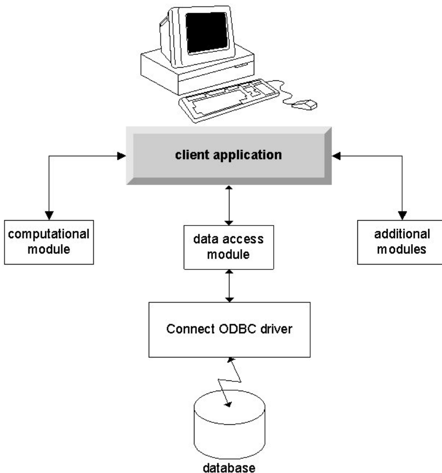
Рисунок 2. Connect ODBC в режиме локального анализа
