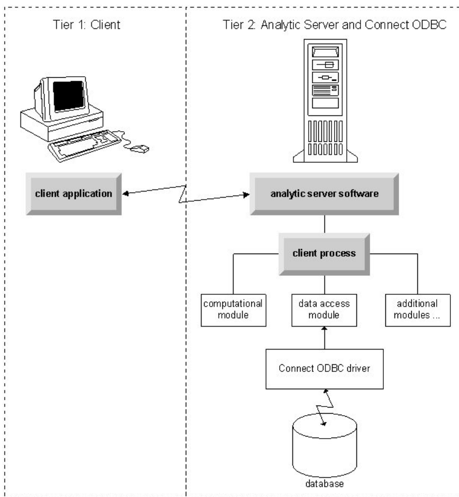
Рисунок 1. Connect ODBC в режиме распределенного анализа
