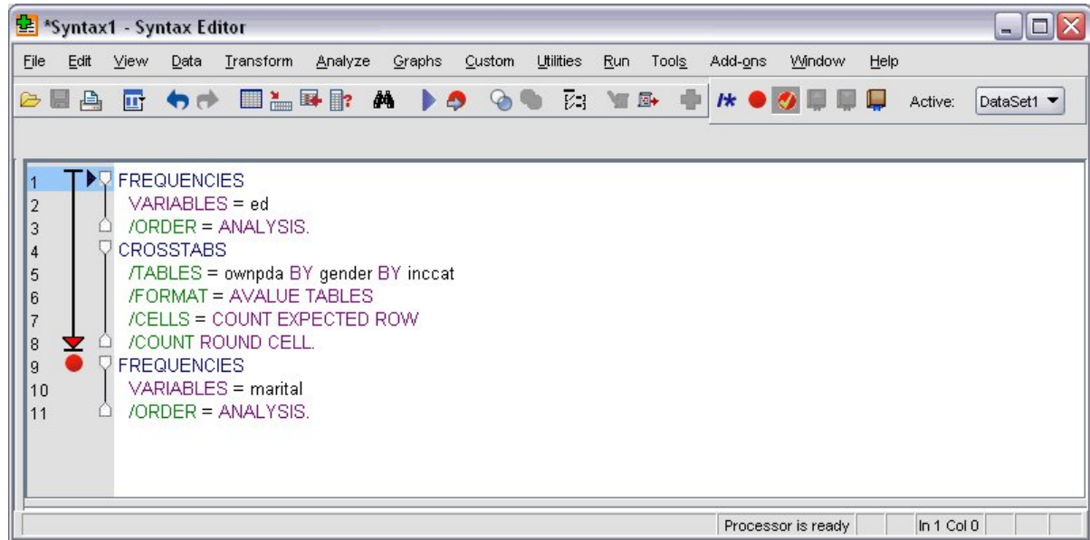
Figure 72. Exécution interrompue à un point de rupture
