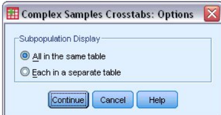
Abbildung 7. Dialogfeld "Optionen"
