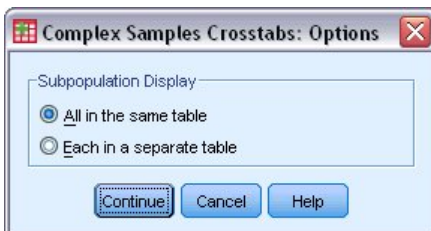
Abbildung 4. Dialogfeld "Optionen"
