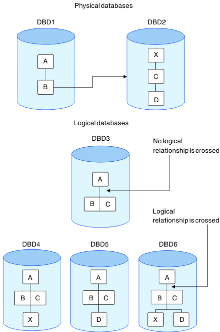
図 96. 論理関係の交差の定義
