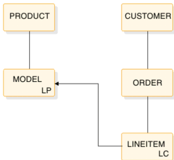
図 167. 単一方向論理関係の例
