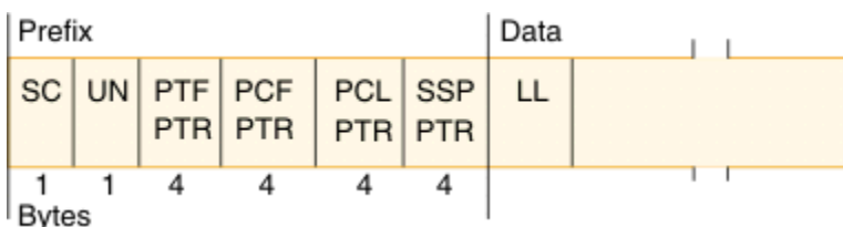
図 63. 直接従属セグメントのフォーマット
