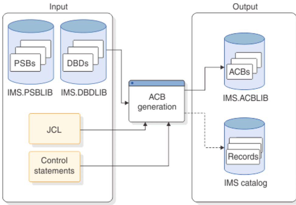
図 235. ACB 生成処理
