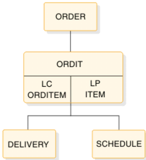
図 95. シンボリック・ポインターを使用する単一方向関係のための論理データ構造
