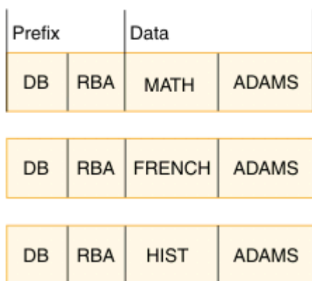
図 179. 受講者ごとのソース・セグメントの例
