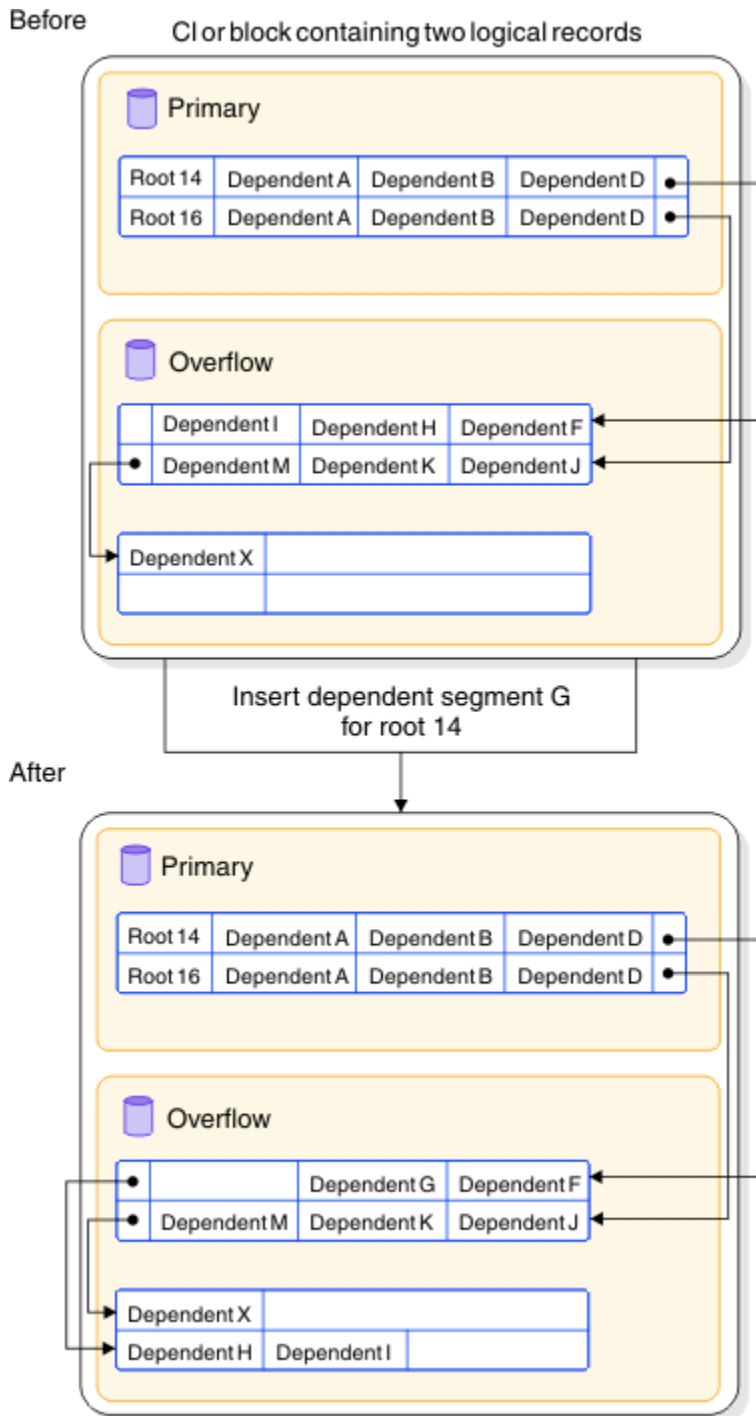
図 30. HISAM データベースへの従属セグメントの挿入 (論理レコードの中にスペースが存在しない場合)
