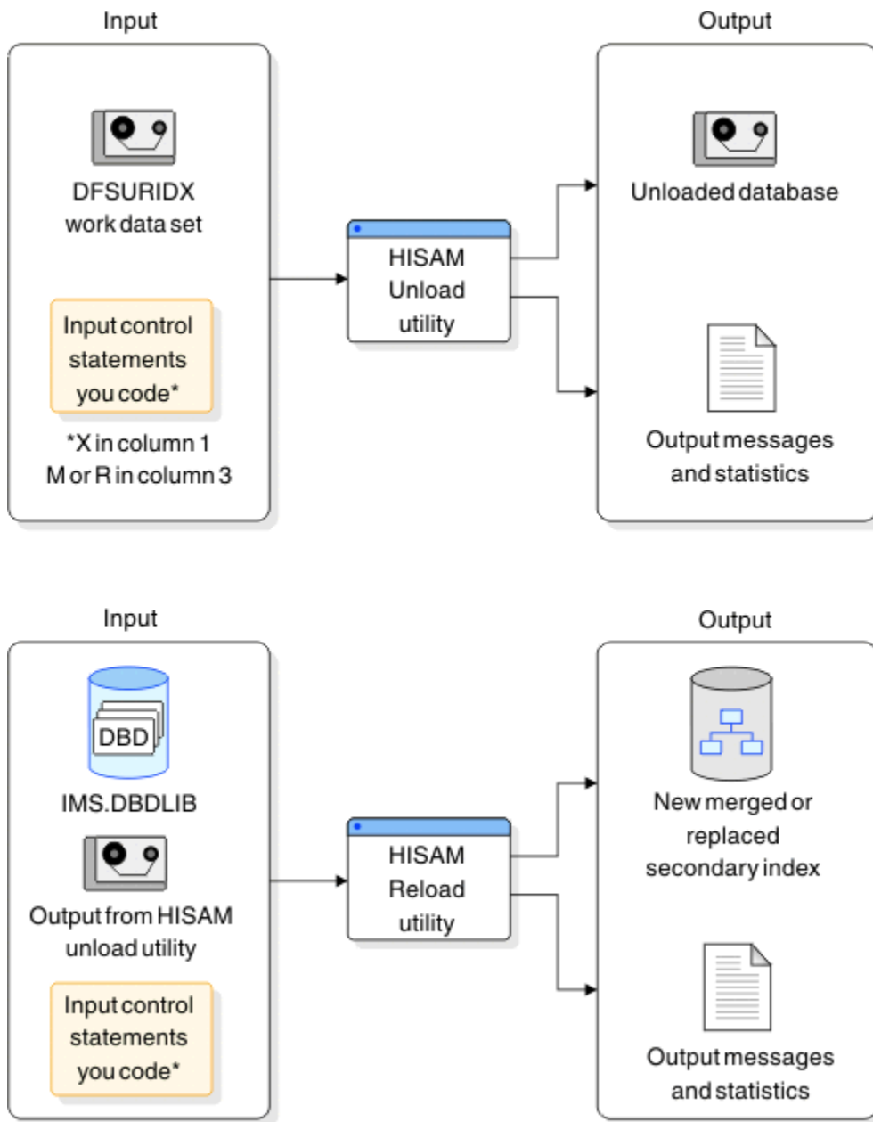
図 258. 副次索引の作成、マージまたは置き換え操作に使用される HISAM 再編成アンロードおよび再ロード・ユーティリティ
