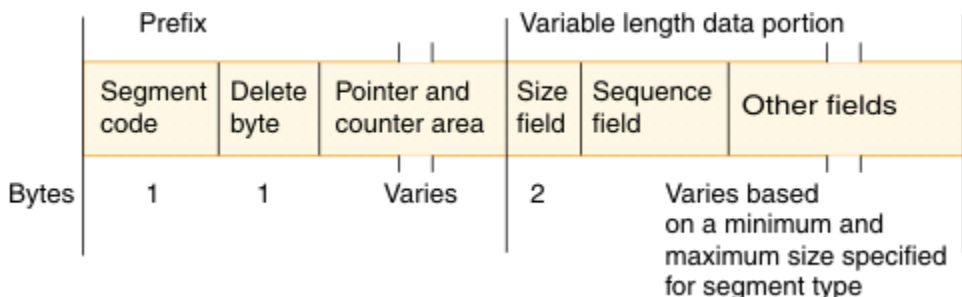
図 10. 可変長セグメントのフォーマット
