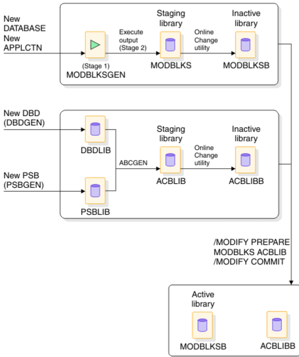
図 289. オンライン変更によるデータベースの追加
