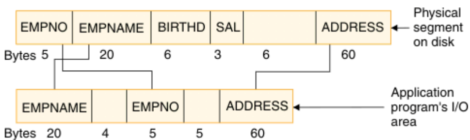
図 199. フィールド・レベル・センシティブティエーのための DBD および PSB コーディング
