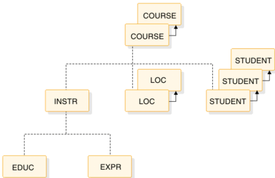
図 42. 物理兄弟順方向ポインター
