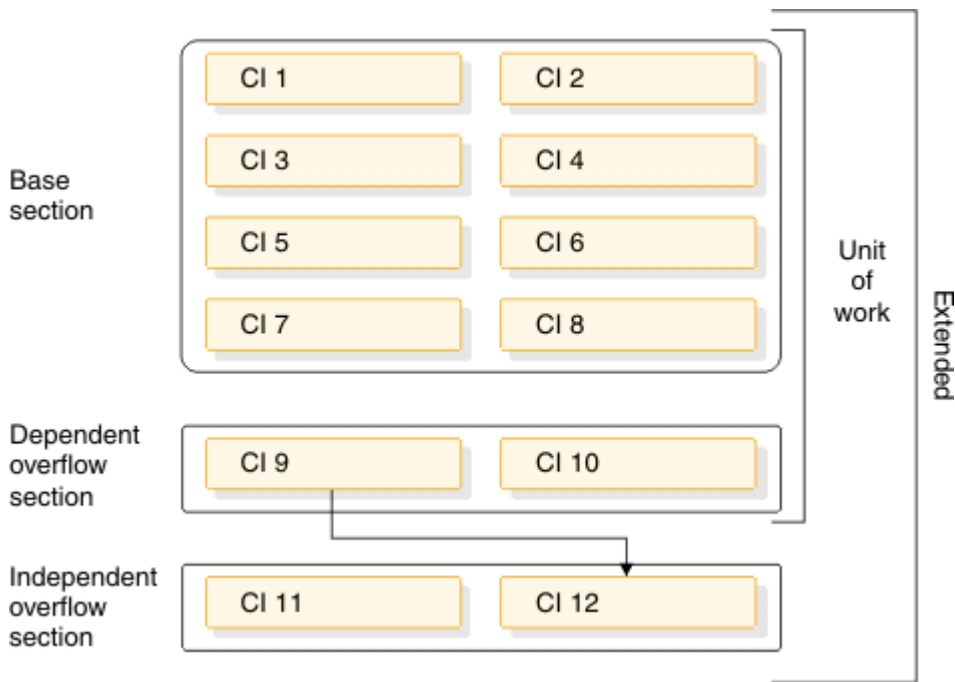
図 65. 独立オーバーフローを使用する UOW の拡張
