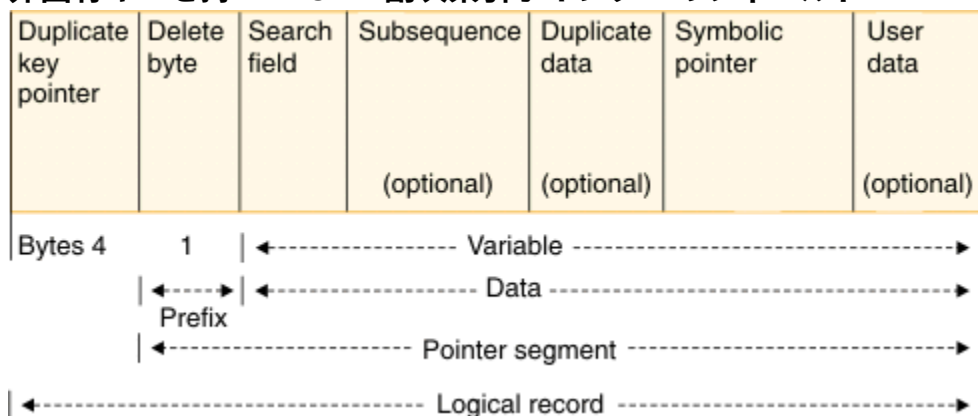
図 184. 非固有キーを持つ HISAM 副次索引ポインタの例
