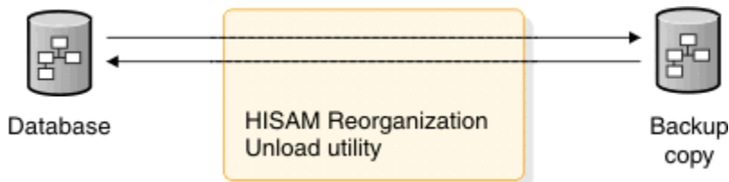
図 243. HISAM アンロードでのバックアップ・コピーの作成
