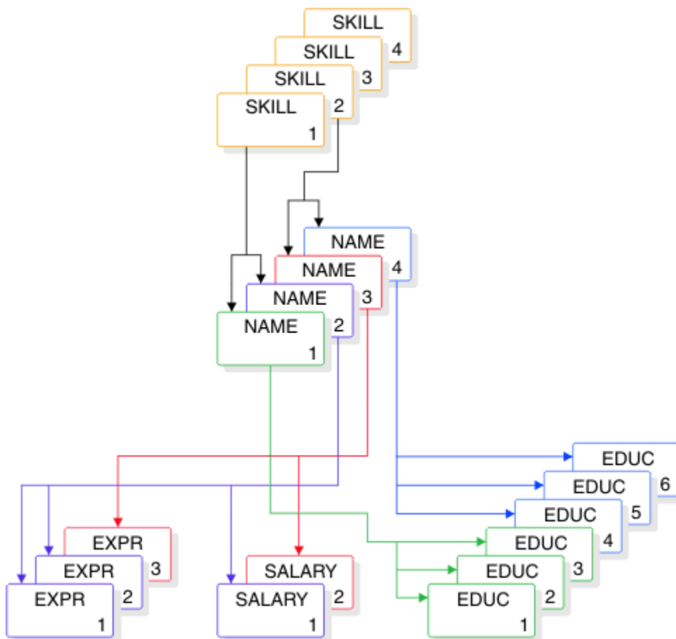
図 24. HISAM データベース・レコードの例
