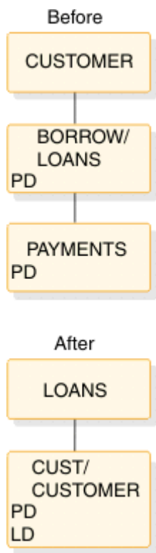
図 147. 論理子、物理対 - 物理削除規則または論理削除規則の例: 削除前および削除後
