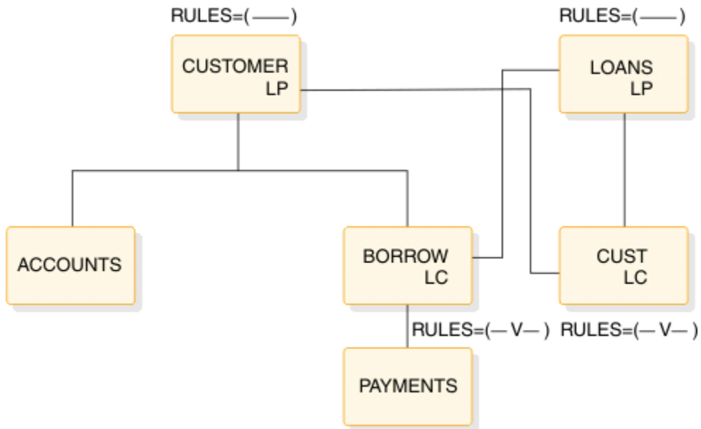
図 151. 論理子、物理対 - 仮想削除規則の例
