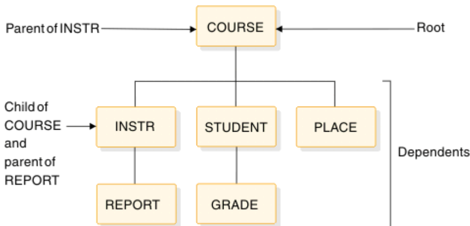
図 1. 学校用データベース・レコードの中のセグメント・タイプ
