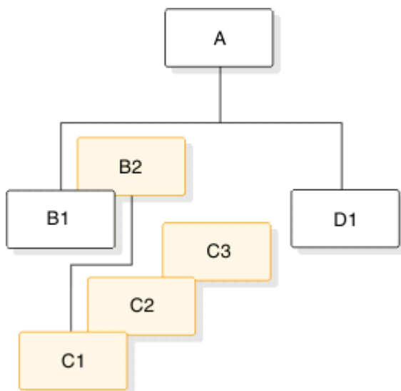
図 31. データベース上の階層セグメントのレイアウト
