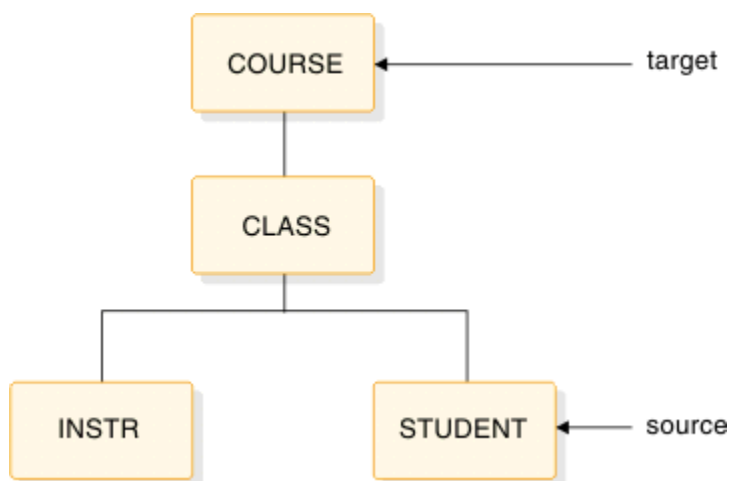
図 186. 副次索引用のソースおよびターゲットを示すデータベース・レコード
