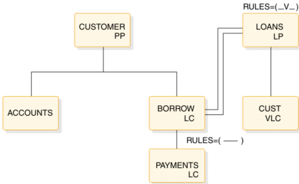
図 130. 論理親、仮想対 - 仮想削除規則の例
