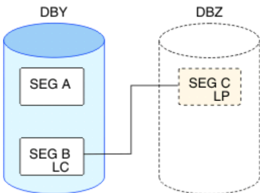
図 279. DBY が存在し、DBZ を追加する
