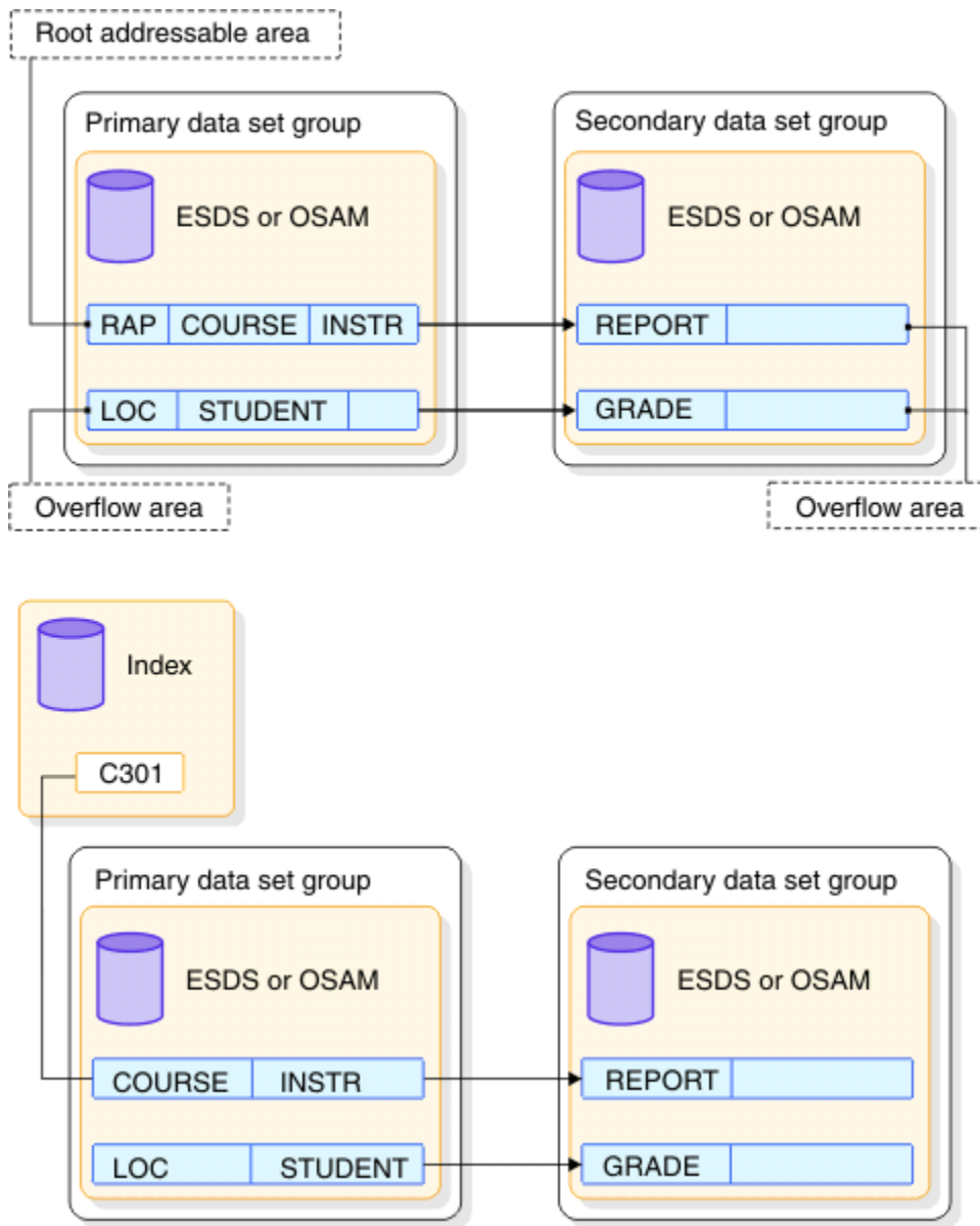
図 213. 複数データ・セット・グループを用いたときのストレージ内の HD データベース・レコード
