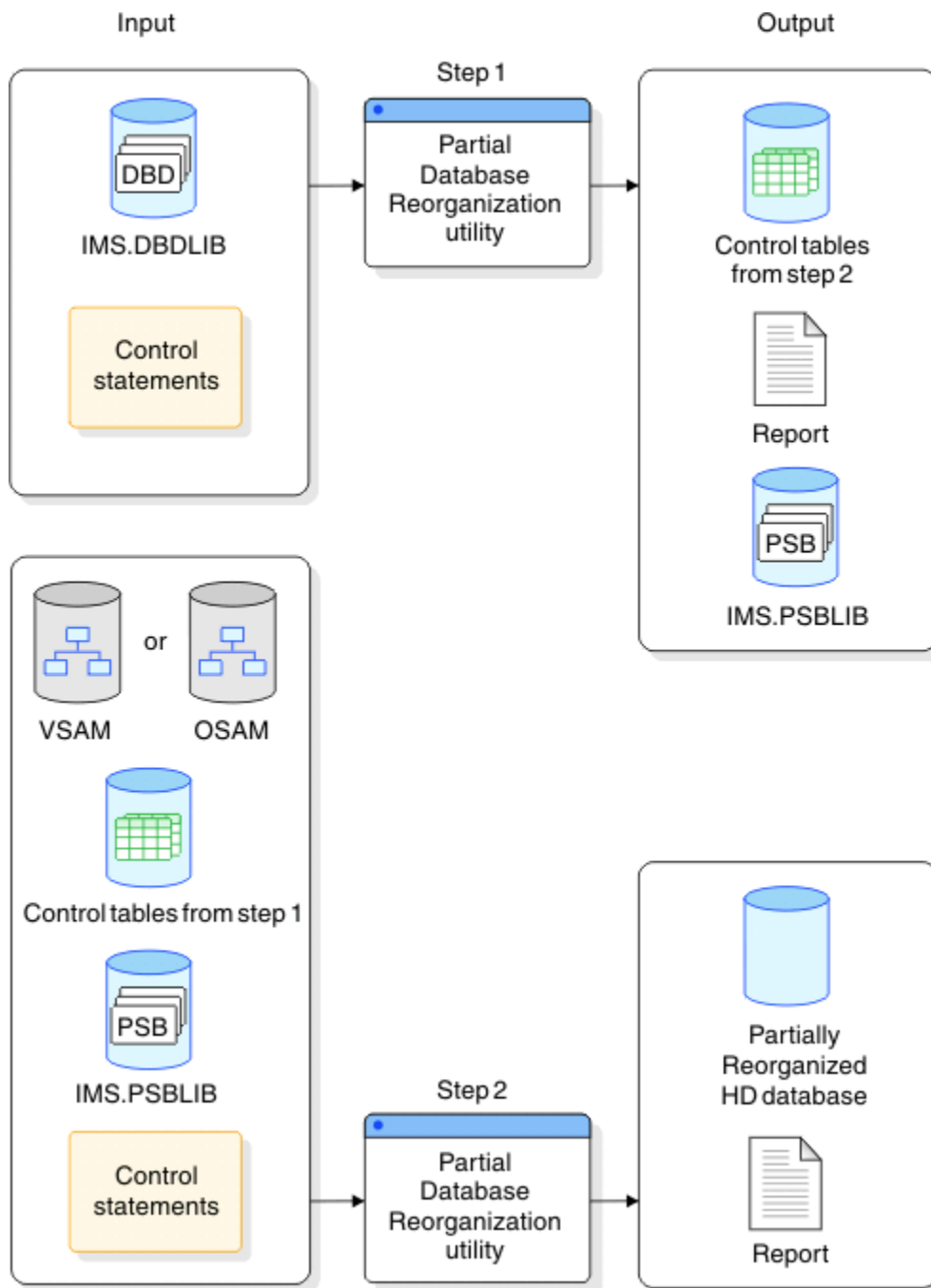
図 261. データベース部分再編成ユーティリティ (DFSPRCT1)
