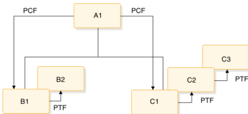
図 56. PCF ポインターと PTF ポインターを使用した場合の従属セグメントの調べ方
