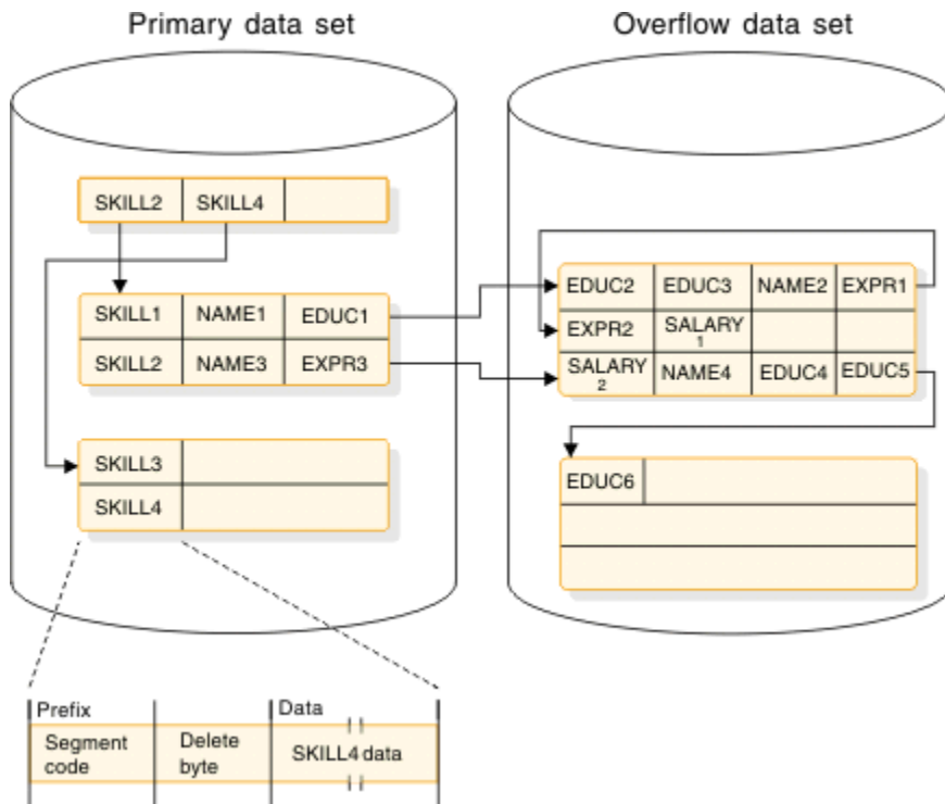
図 25. ストレージの中の HISAM データベース・レコードの例
