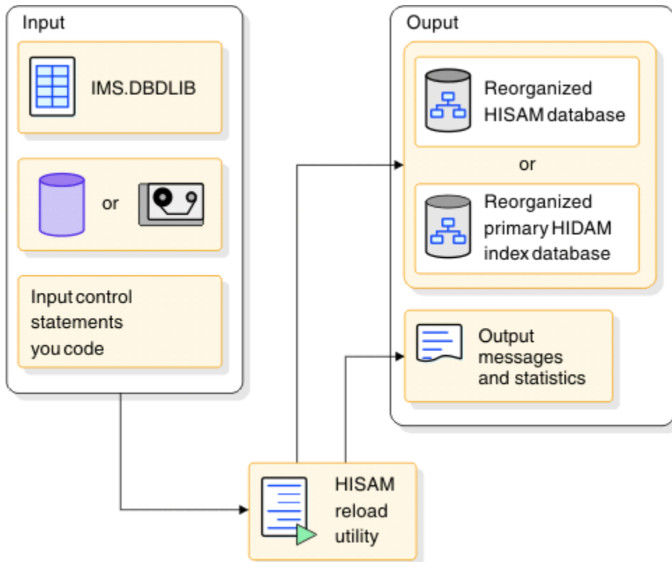
図 251. HISAM 再編成再ロード・ユーティリティ (DFSURRLO)
