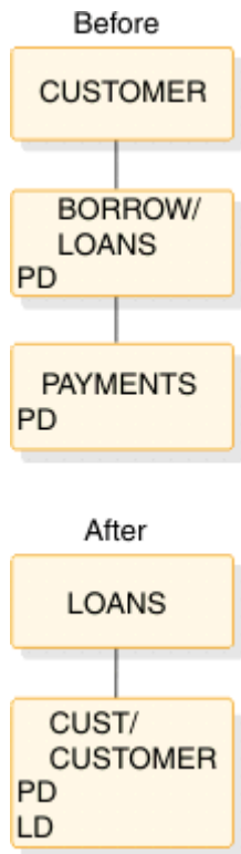
図 144. 論理子、仮想対 - 論理削除規則の例: 削除前および削除後
