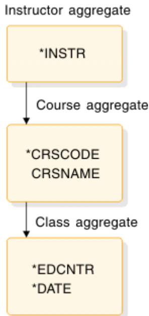
図 219. インストラクター・スケジュールの概念的なデータ構造
