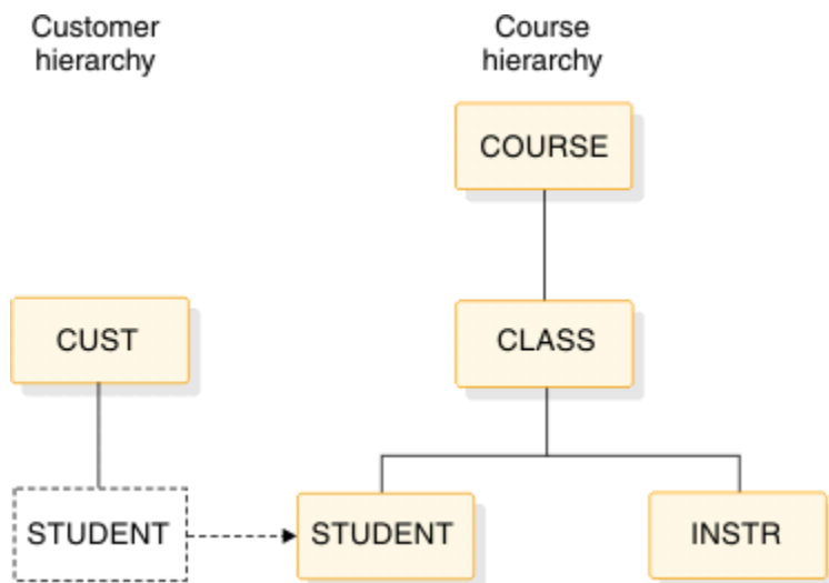
図 221. 教育用階層
