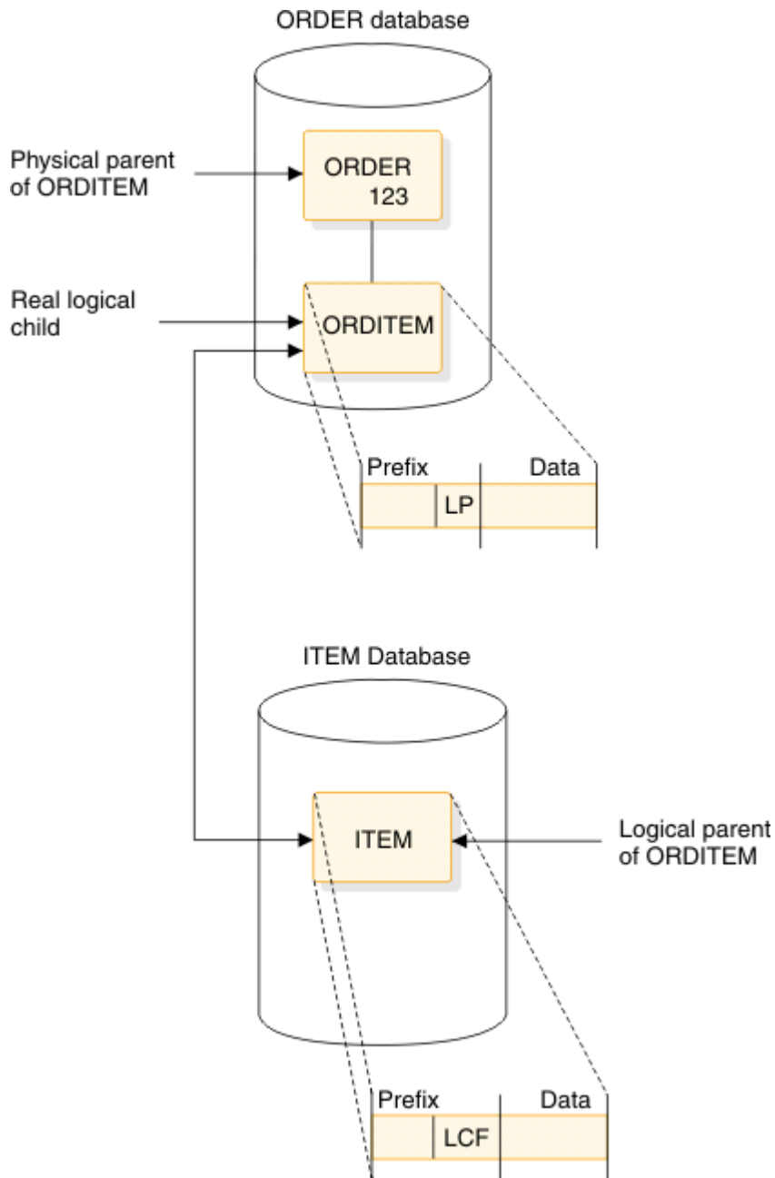
図 80. 論理第 1 子 (LCF) ポインター (仮想対の論理関係においてのみ使用)
