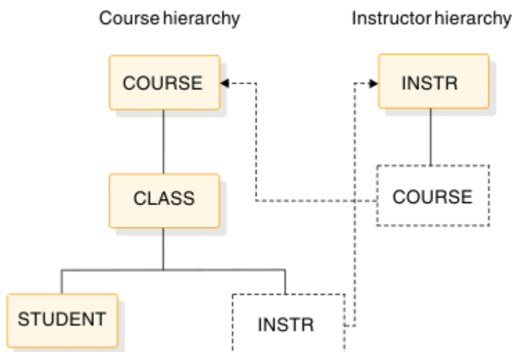
図 222. 両方向論理関係
