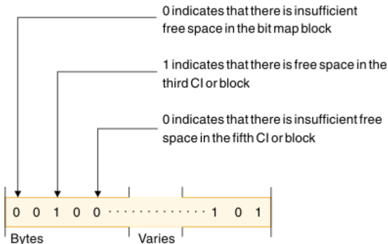
図 46. HD データベースのビットマップ
