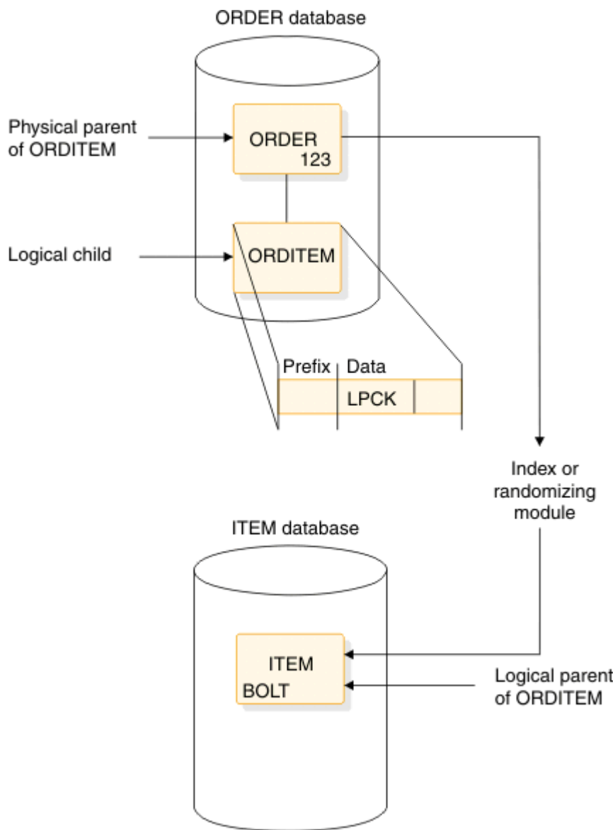
図 79. 記号論理親 (LP) ポインター
