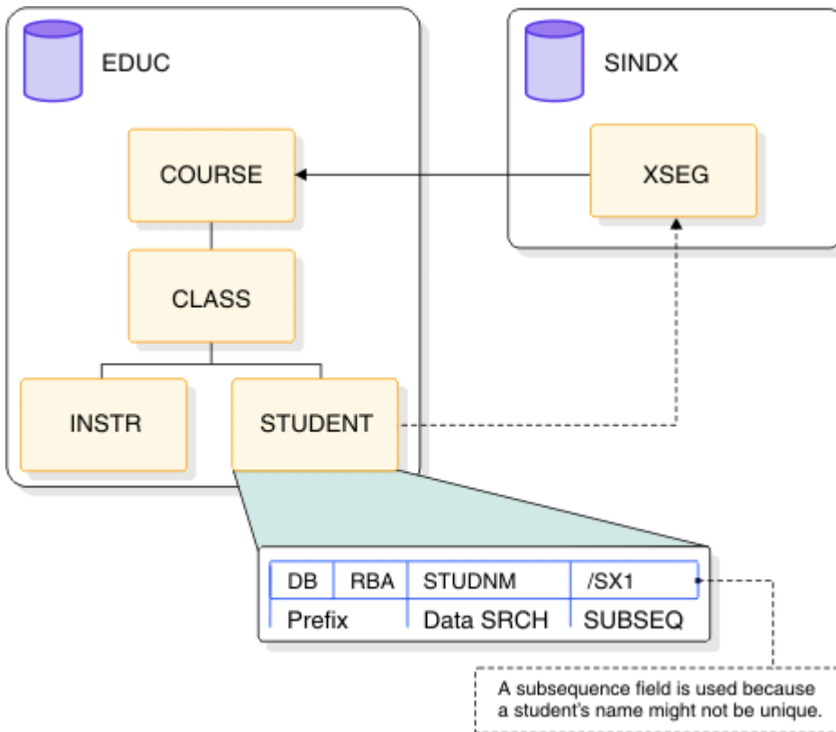
図 194. 副次索引の例でのデータベース
