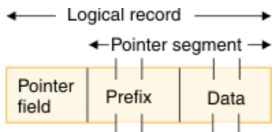
図 180. ポインター・セグメントが入っている論理レコードの例
