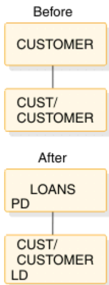
図 125. 論理親、仮想対 - 論理削除規則の例: 削除前および削除後
