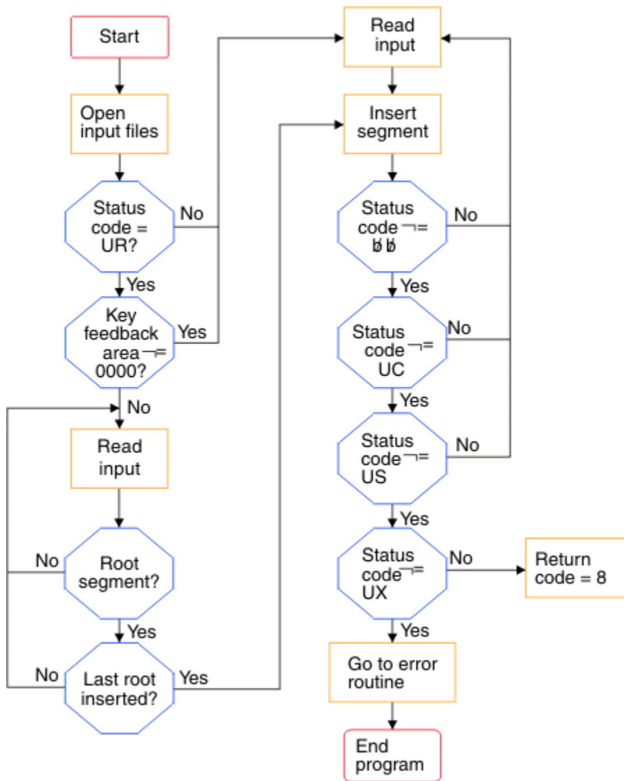
図 242. 再始動可能初期ロード・プログラムの論理
