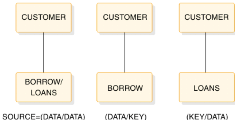
図 164. 連結セグメントの関係
