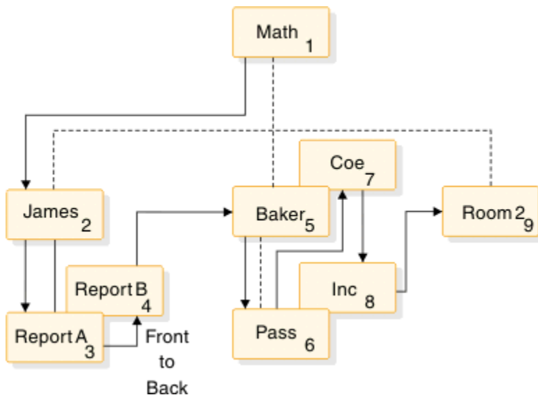
図 4. 学校用データベースのセグメント・オカレンスの階層順
