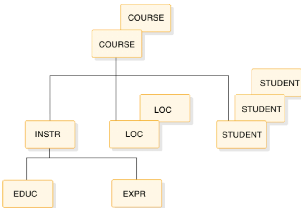
図 36. ポインタの図のためのデータベース・レコードの例
