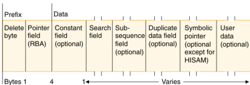
図 182. 副次索引の中のポインター・セグメントのフィールド
