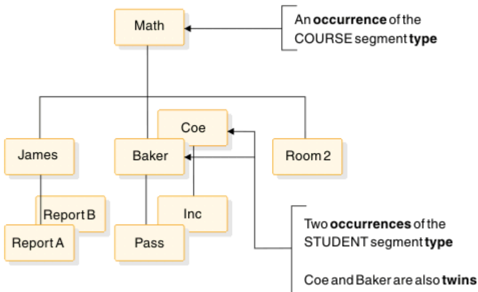
図 2. 学校用データベース・レコードの中のセグメント・オカレンス
