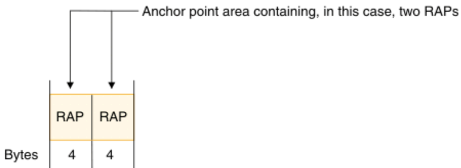
図 49. HDAMまたはPHDAMのアンカー・ポイント域
