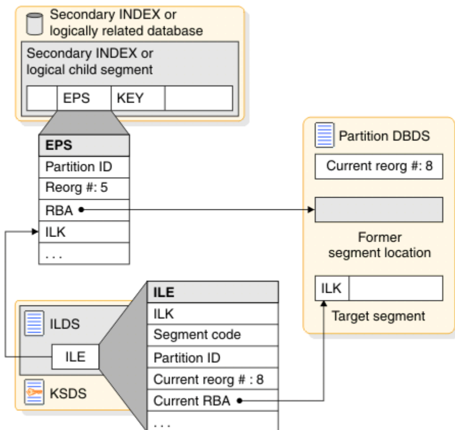
図 268. 再編成後の HALDB ポインター
