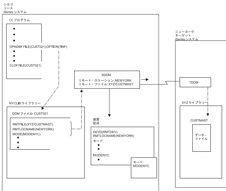
図 11. DDM ファイル・パラメーターとシステムとの関係
