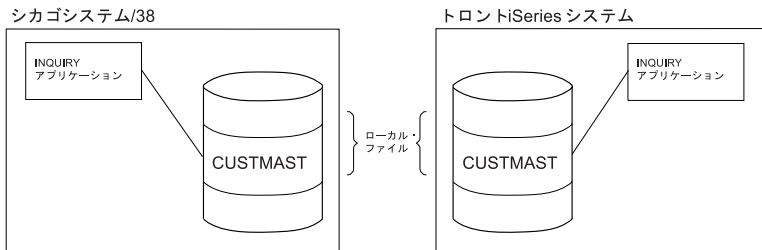
図 40. ローカル照会を行う 2 つの非 DDM サーバー
