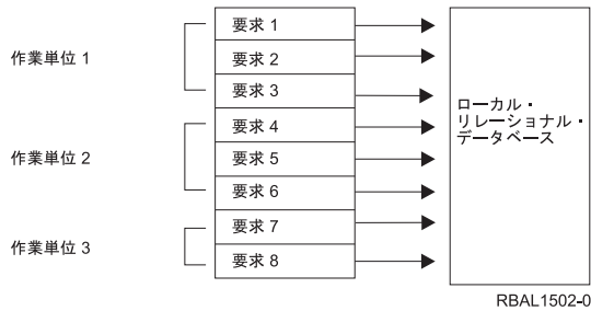
図3. ローカル・リレーショナル・データベースにおける作業単位
