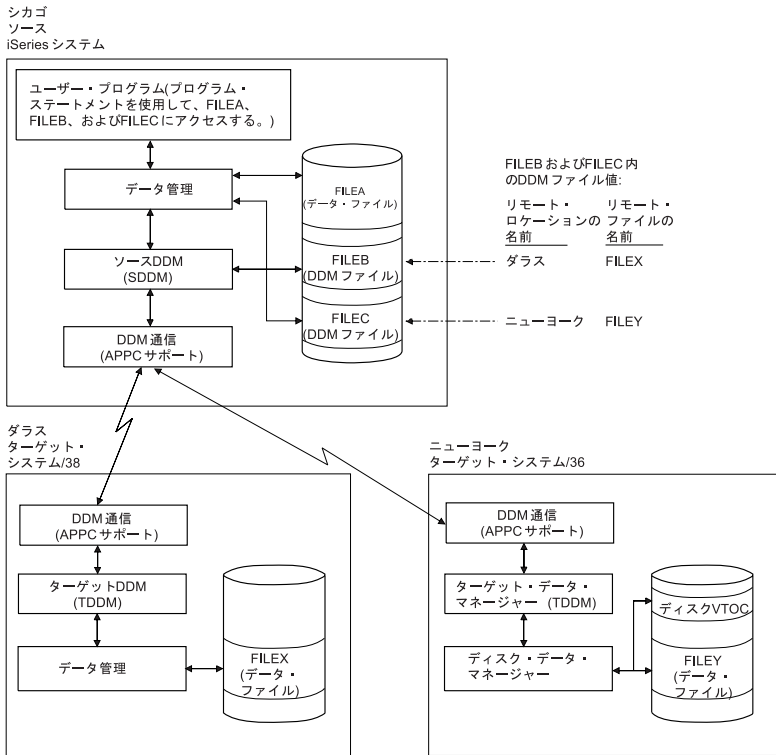
図 17. 例: 複数のローカルおよびリモート・ファイルへのアクセス: システム/38 およびシステム/36 との通信リンクを持った IBM i。
