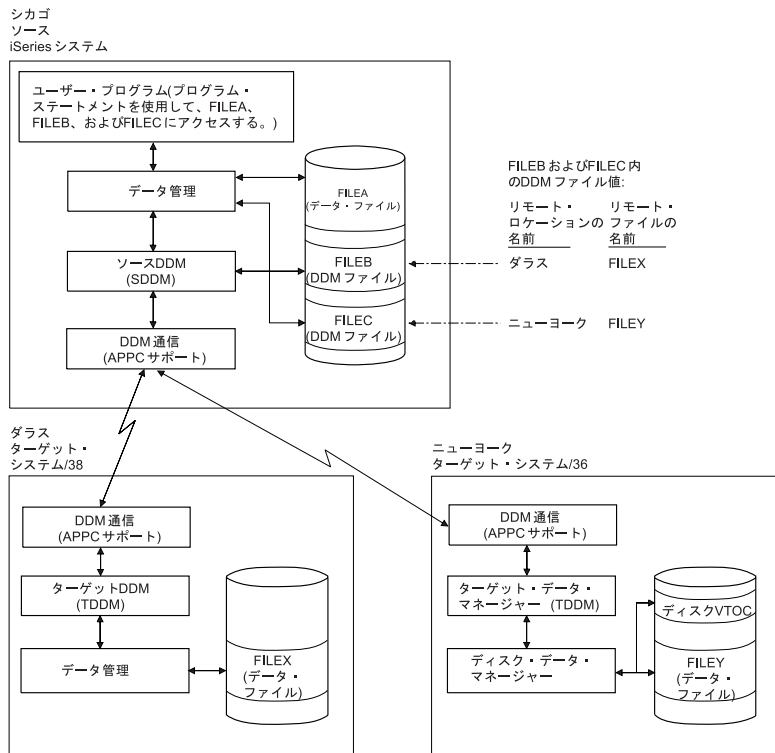
図 18. 例: 複数のローカルおよびリモート・ファイルへのアクセス: システム/38 およびシステム/36 との通信リンクを持った IBM i。
