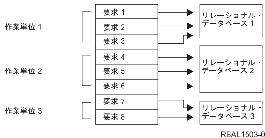
図4. 分散リレーショナル・データベースにおけるリモート作業単位
