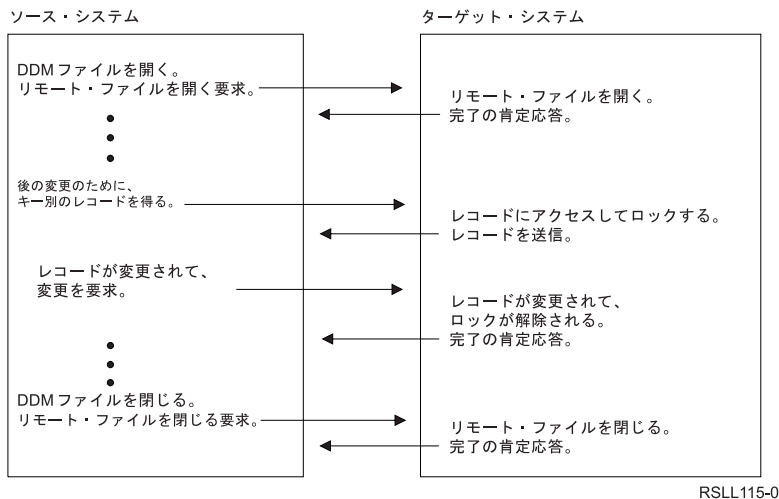
図 14. 入出力操作要求の一般的処理法
