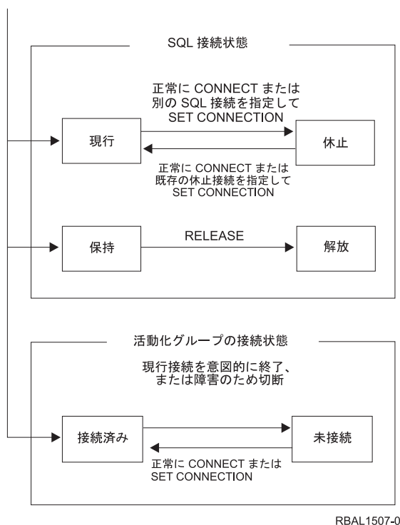
図 24. アプリケーションが指定する分散作業単位接続および活動化グループの接続の状態遷移
