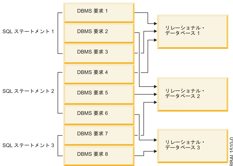
図 6. 分散リレーショナル・データベースの分散要求
