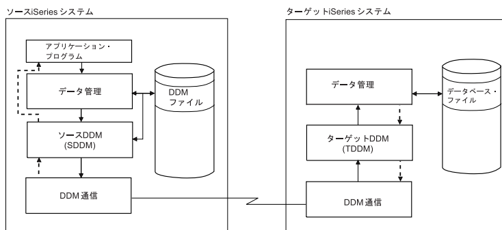
図 10. DDM を用いた通信
